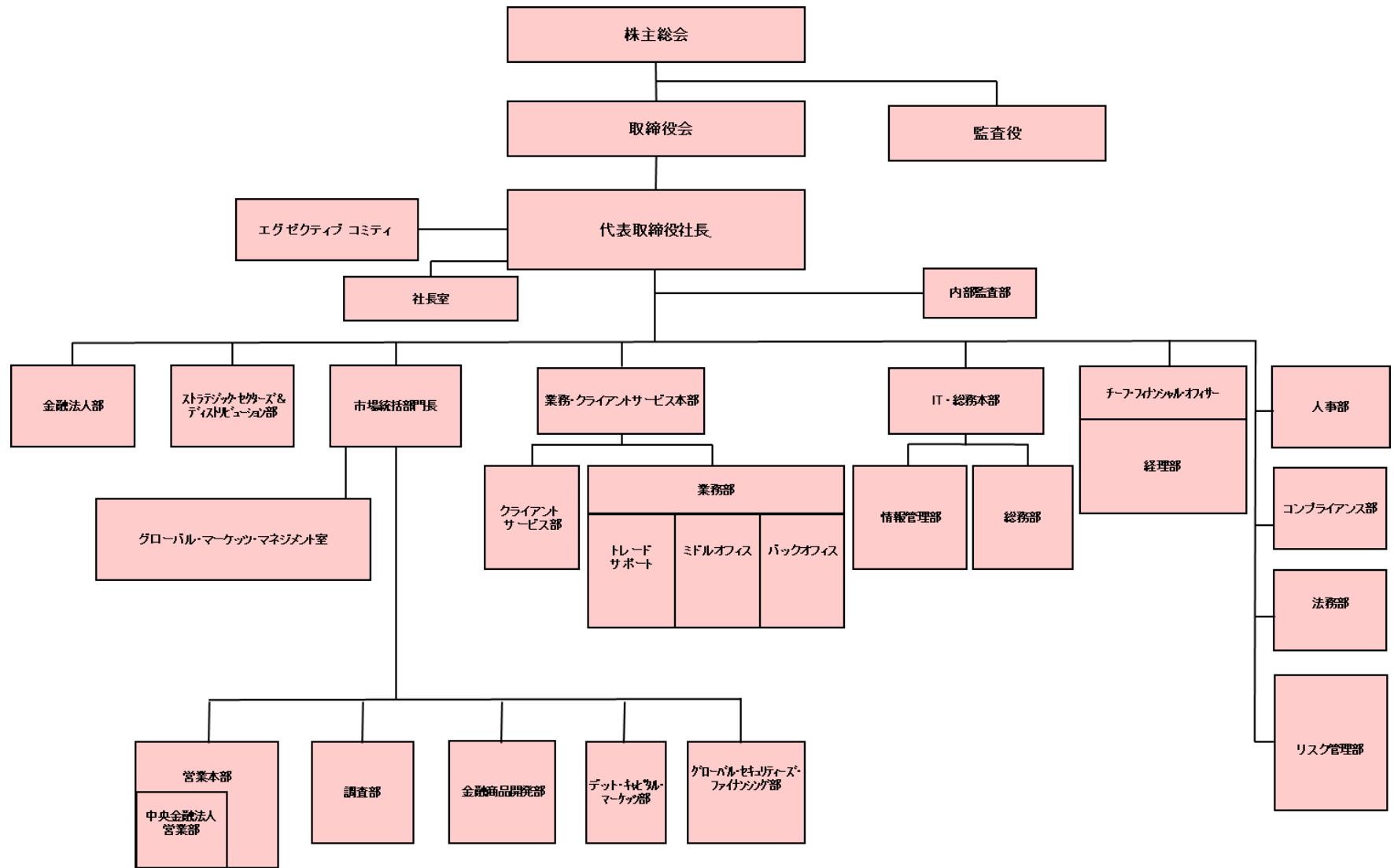
(会社組織図)
